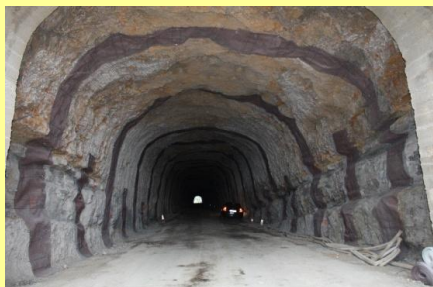
Inici de la restauració. Anivellació de les roques per al seu encofrat
